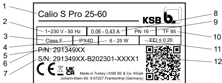
Bild 1: Märkskylt (exempel)
