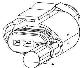
Bild 17: Demontera kontakten
