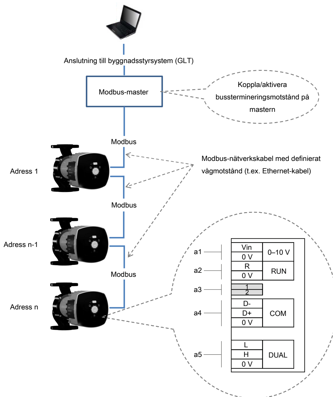
Bild 15: Modbus-kabelanslutning pumpaggregat
