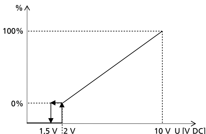
Bild 30: Analog signal 0-10 V som börvärdesinställning på pumpaggregatet
