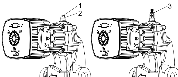
Bild 8: Montera avluftningsskruv för horisontellt monteringsläge
