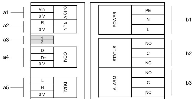
Bild 33: Elektriskt anslutningsschema
