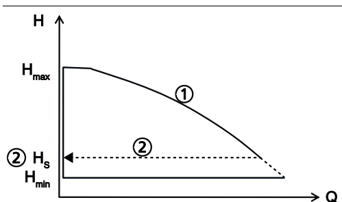
Bild 22: Funktion konstant tryckreglering
