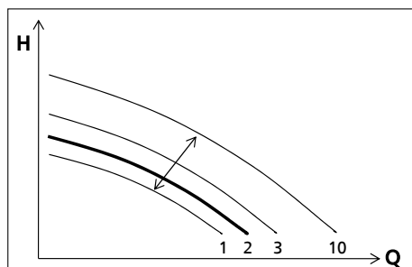
Bild 28: Funktion termostatdrift, drift på varvtalssteg 2
