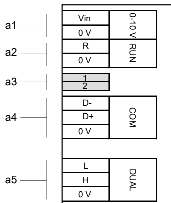
Bild 18: Plintschema dubbelpumpdrift
