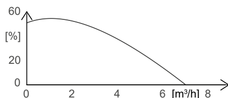
Bild 27: Besparingspotential för Eco-Mode jämfört med proportionellt tryck med modellstorlek 25-100 som exempel
