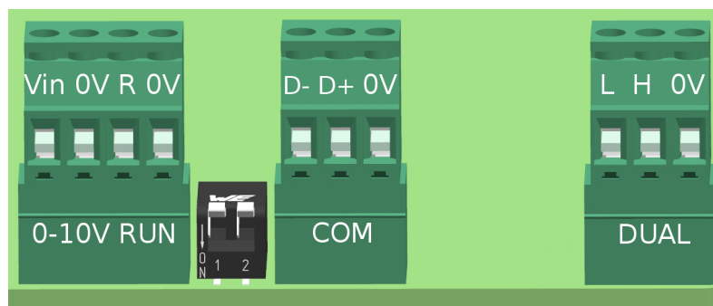
Bild 17: Plintschema
