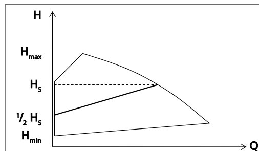
Bild 24: Funktion proportionell tryckreglering
