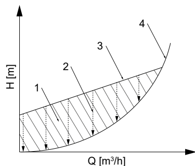
Bild 31: Den dynamiska styrningens princip
