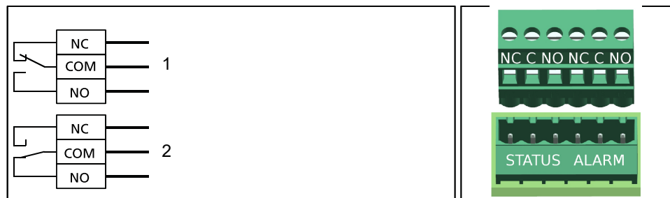
Bild 11: Elektriskt anslutningsschema driftmeddelande
