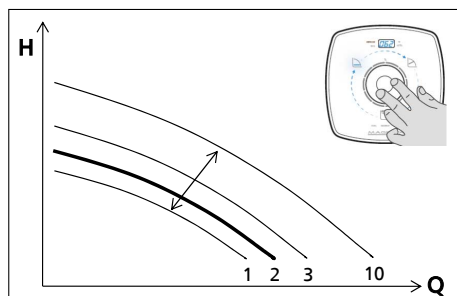
Bild 29: Inställning termostatdrift
