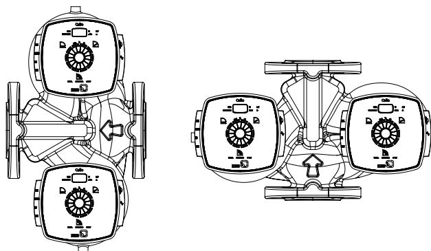
Bild 7: Tillåtna monteringslägen
