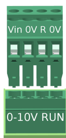
Bild 13: Plintpar 0-10 V
