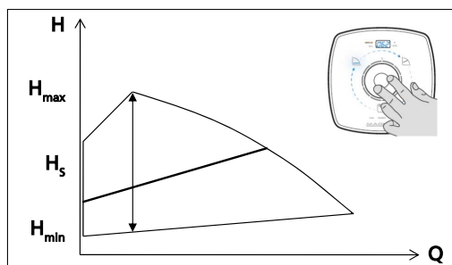
Bild 25: Inställning proportionell tryckreglering
