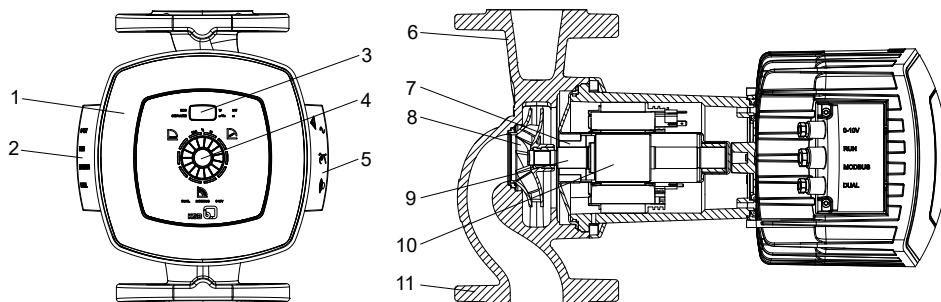
Bild 5: Illustration av pumpaggregat
