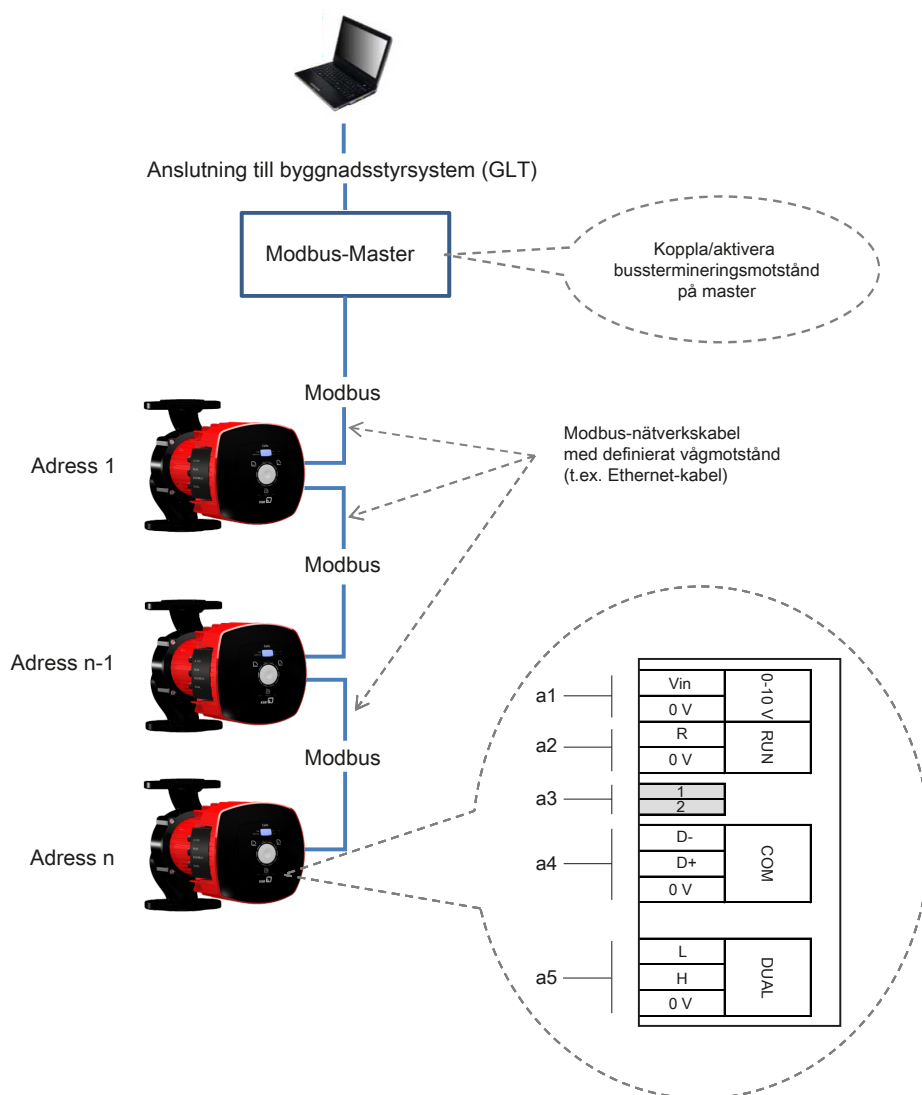
Bild 13: Modbus-kabelanslutning pumpaggregat
