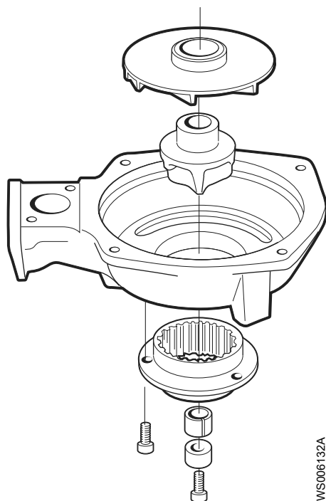
Figur 18: M-pumphjul
