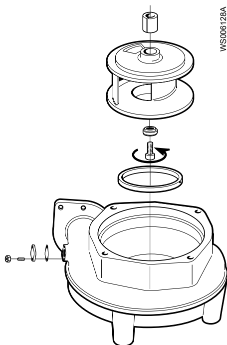
Figur 13: C-pumphjul
