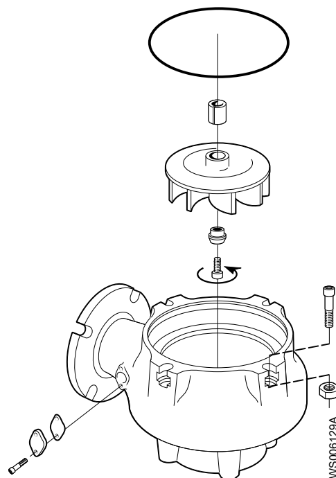
Figur 14: D-pumphjul
