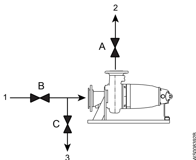
Figur 19: Ventilerna A-D för T-installation (generell pump visas)
