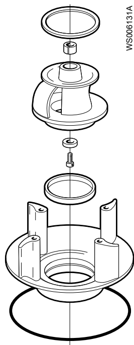
Figur 15: L-pumphjul
