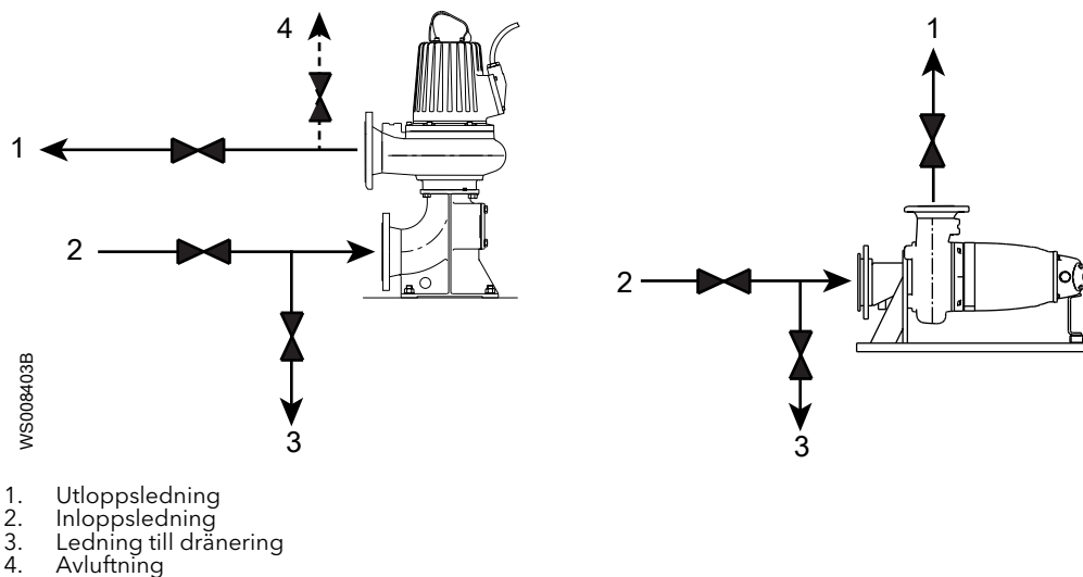
Figur 6: Avstängnings- och avluftningsventiler för T- och Z-installation (generella pumpar visas)
