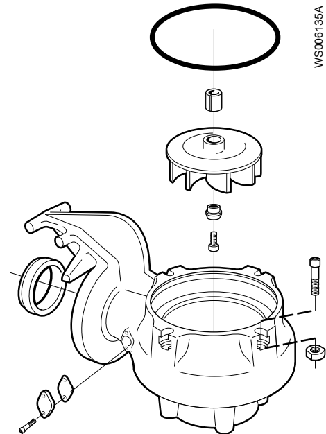
Figur 14: D-pumphjul
