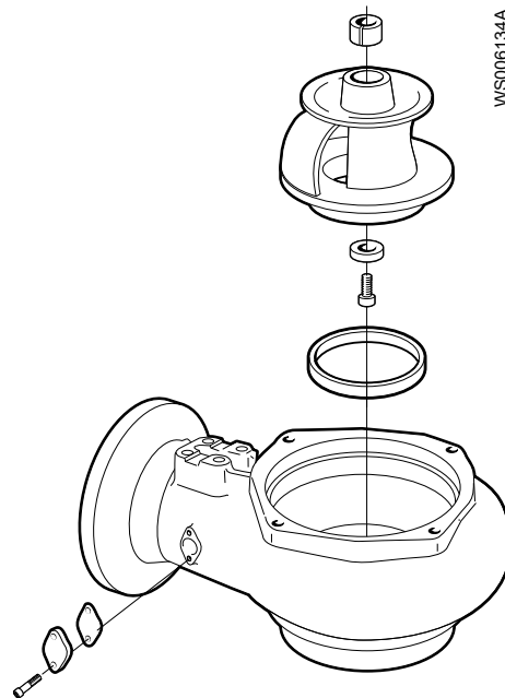
Figur 13: C-pumphjul
