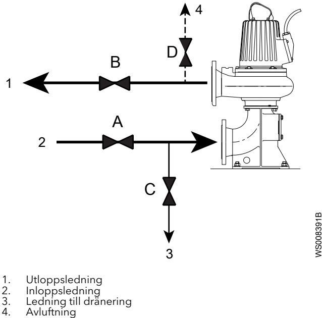
Figur 19: Ventilerna A-D för T-installation (generell pump visas)
