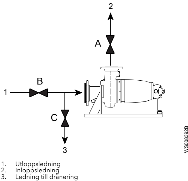
Figur 20: Ventilerna A-C för Z-installation (generell pump visas)
