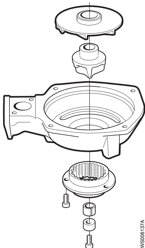
Figur 18: M-pumphjul
