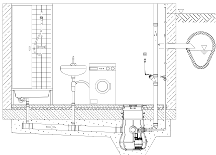
Installationsexempel – enkelpump
