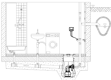
Installationsexempel – dubbelpump
