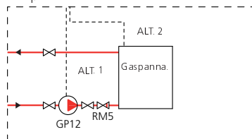
Gaspanna
