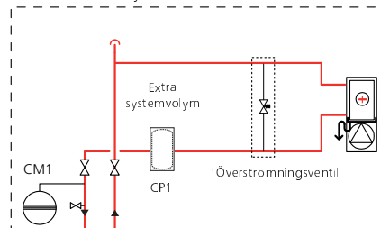
Fläktkonvektorsystem
