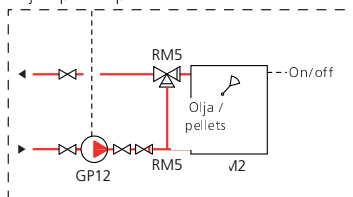
Olje-/pelletsanna
