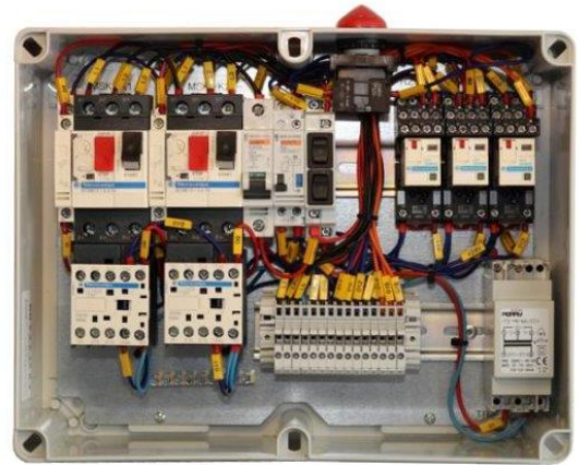
Automatikskåp BN2.
