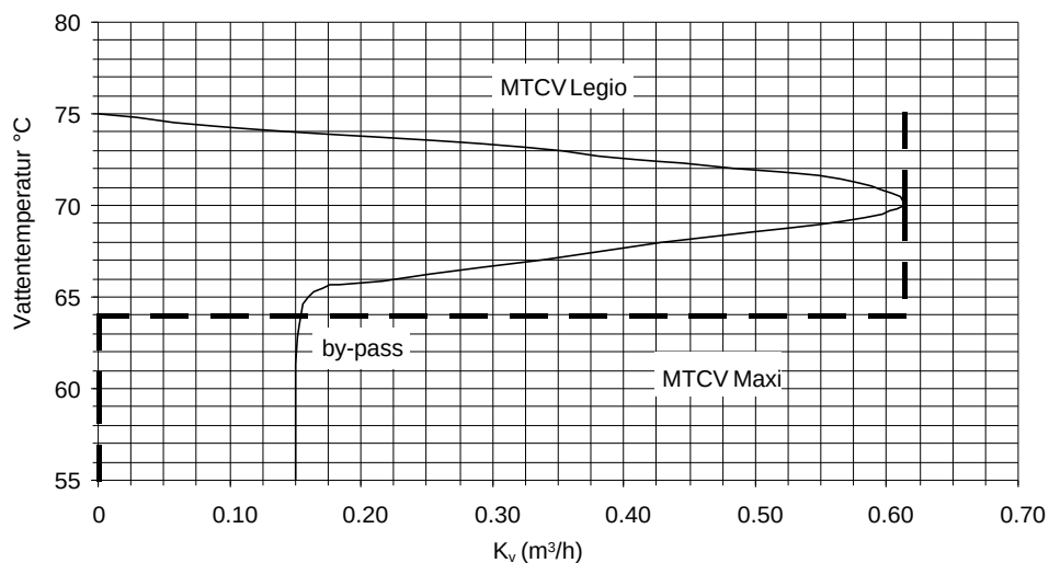
Fig. 22 Desinficeringsprocess - MTCV DN 20
