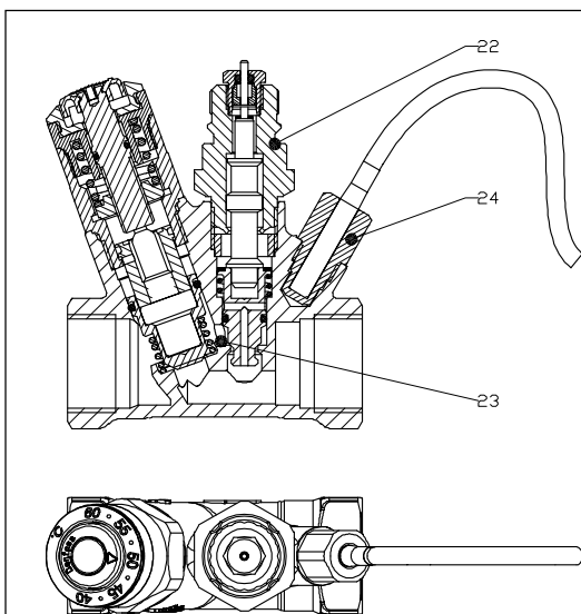
Fig.13 Konstruktion MTCV Maxi
