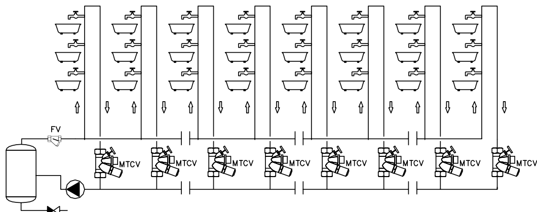
Fig. 8 Principskiss med MTCV Legio
