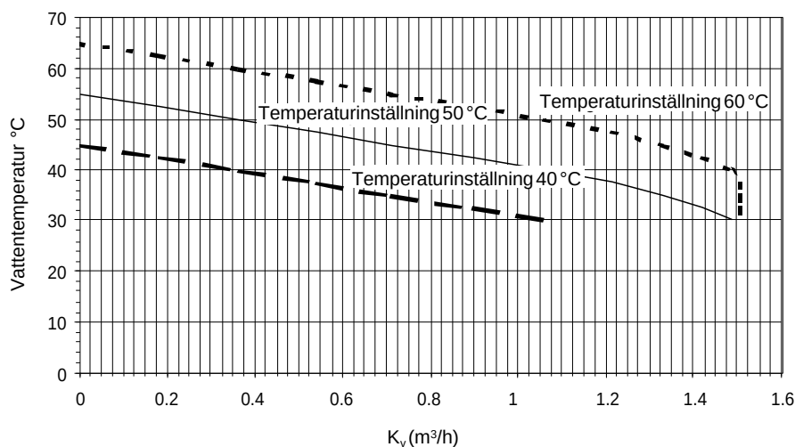
Fig. 16 Temperatur- och k_v -diagram MTCV DN 15
