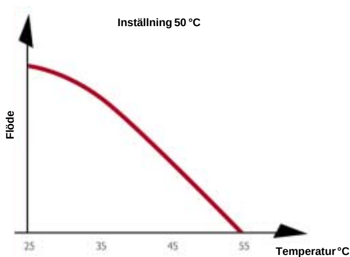
Fig. 7 Reglerprincip MTCV Basic
