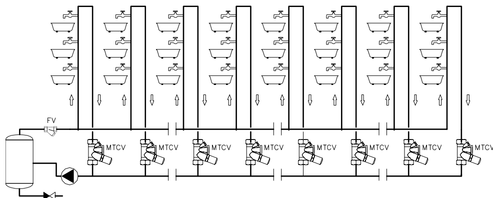
Fig. 6 Principskiss med MTCV Basic
