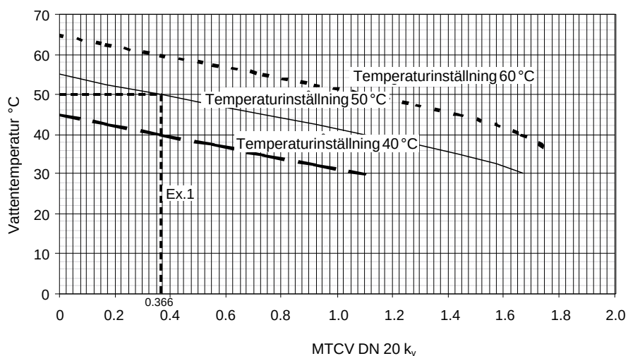
Fig. 18 Temperatur- och k_v -diagram MTCV DN 20
