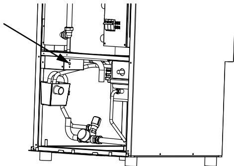
Bild 8 Placering överhettningsskydd
