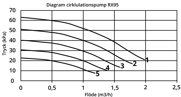
Bild 7 Pumpdiagram
