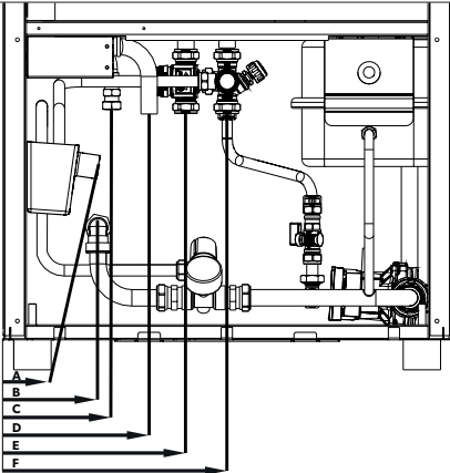
Bild 2 Vattenanslutningar framifrån
