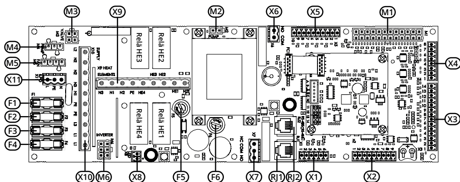
Bild 6 Översikt anslutningar
