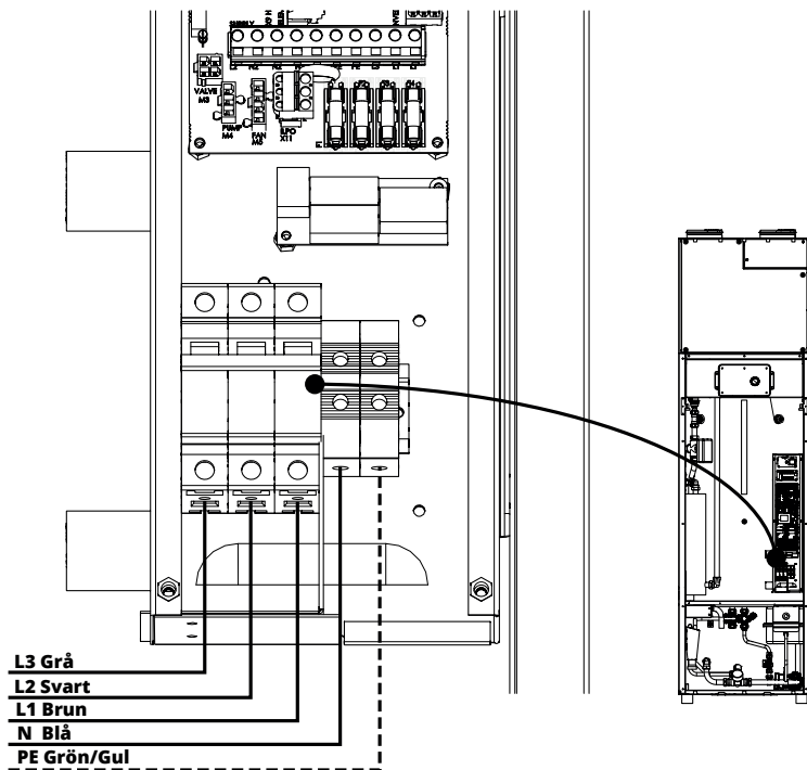
Bild 4 Allpolig brytare och anslutning till automatsäkring
