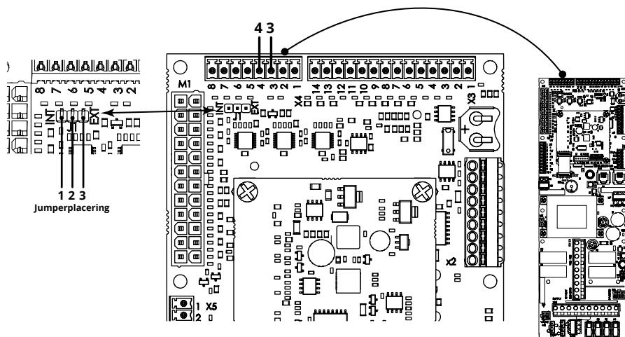
Bild 5 Anslutning mellan extern rumsgivare
