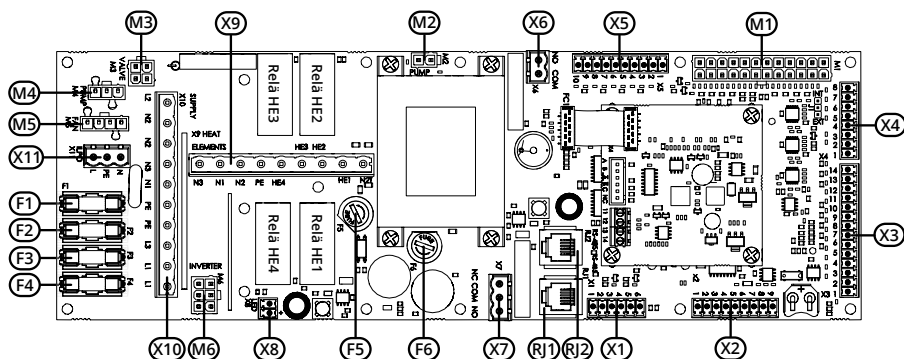
Bild 9 Översikt anslutningar
