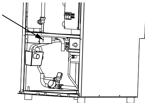
Bild 11 Placering överhettningsskydd
