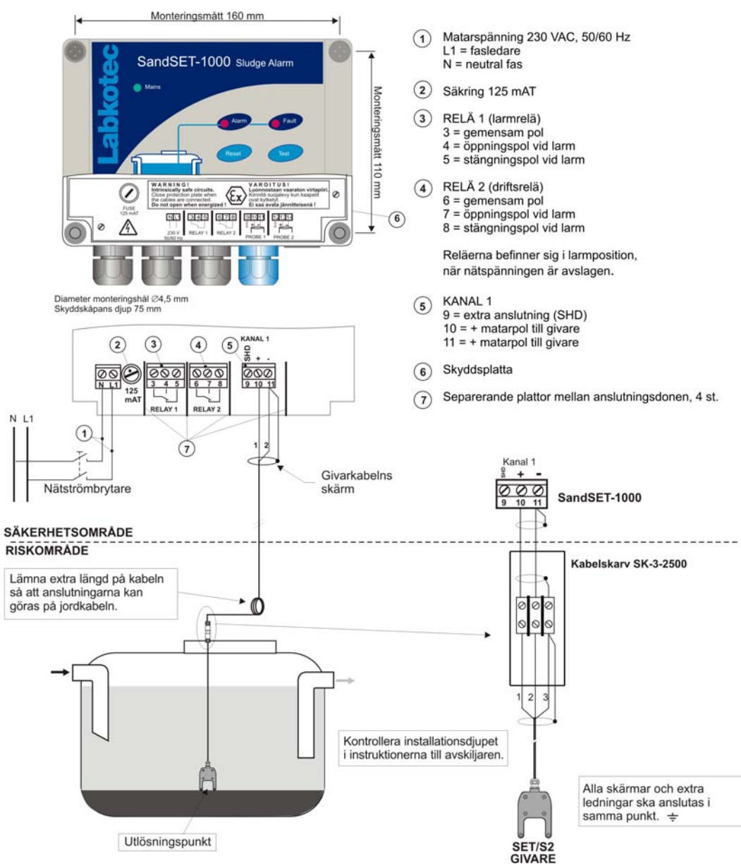
Bild 3. Installation av larmanordning SandSET-1000
