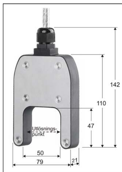
Bild 9. Mått ritning av givaren SET/S2
