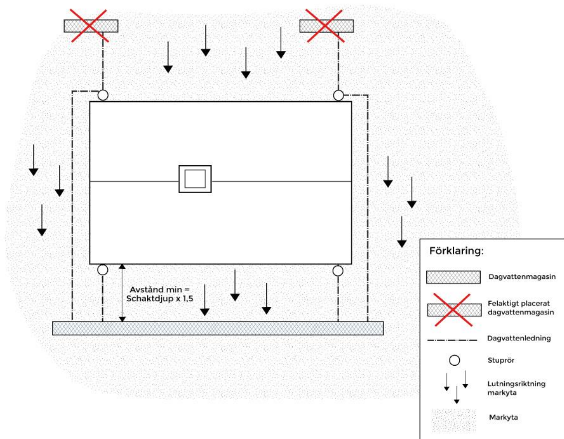
Figur 29. Placering dagvattenmagasin lutande markyta alternativ 2.
