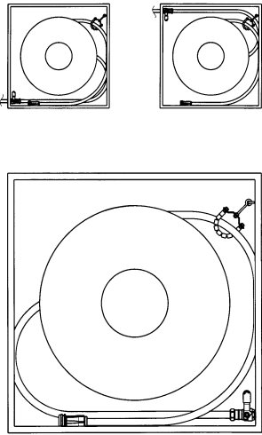
Flexibele montageset, 3 verschillende posities van de afsluiter in de kast mogelijk
