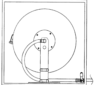
Zwenkarmmontageset gemonteerd in kast
