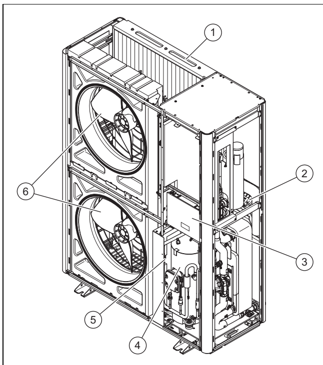
1 Fordamper 2 Printplade INSTALLER BOARD 3 Printplade HMU 4 Kompressor komponenter 5 Komponenter INVERTER 6 Blæser
