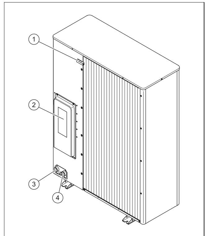
1 Temperatursensor vid luftintaget 2 Skydd för de elektriska anslutningarna 3 Anslutning för värmeter, G 1 1/4" 4 Anslutning för värmeledning, G 1 1/4"
