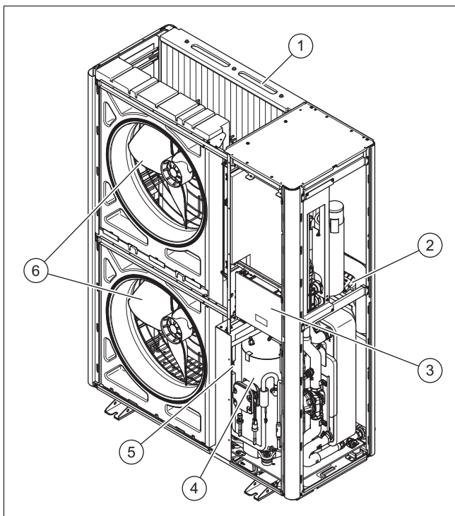
1 Förångare 2 Kretskort INSTALLER BOARD 3 Kretskort HMU 4 Kompressorkomponent 5 Komponentgrupp INVERTER 6 Fläkt
