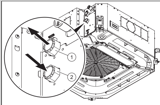
1 Hidraulikus kör visszatérő ága ürítőcsavarral 2 Előremenő hidraulika-kör
