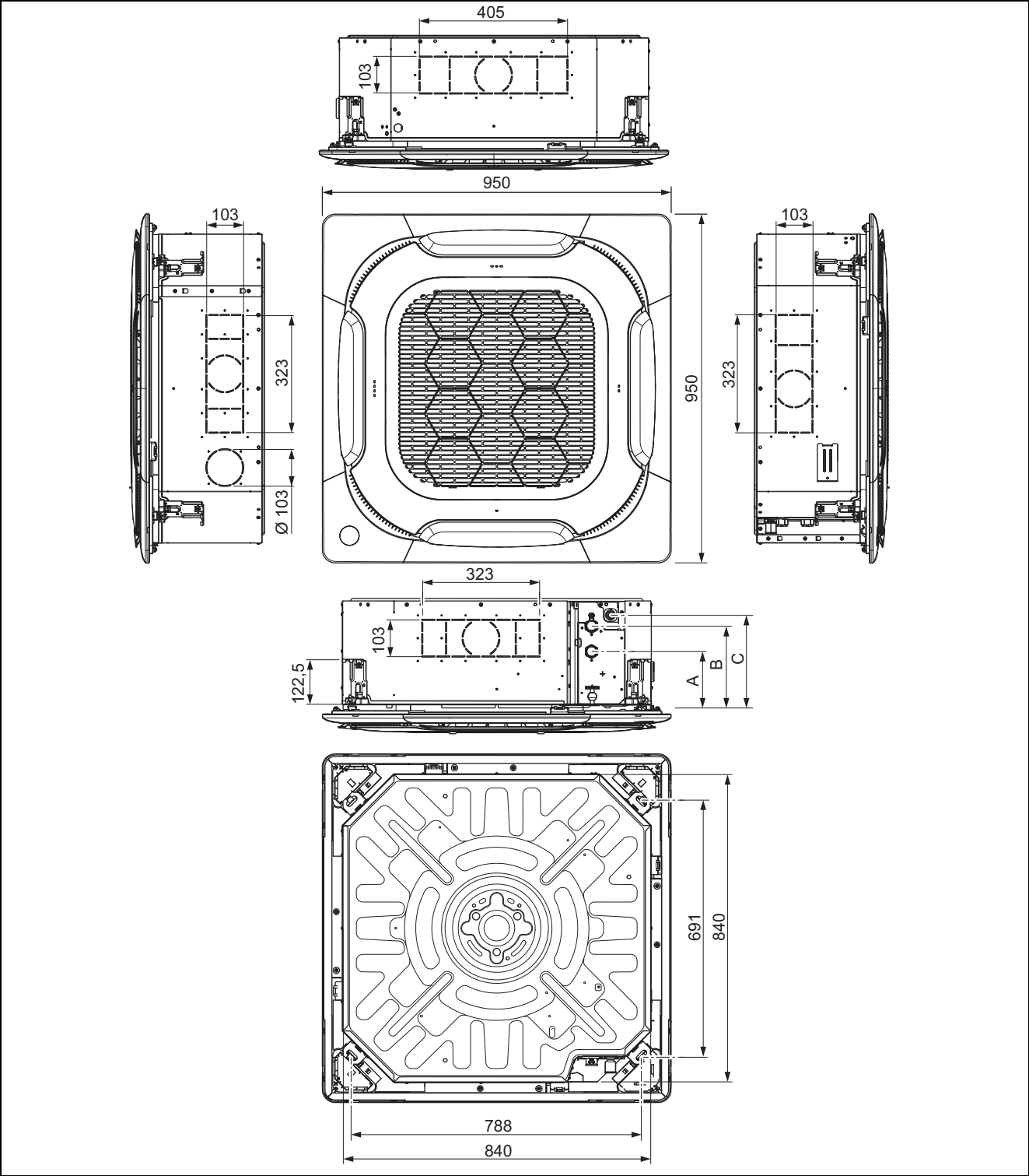
Размери [mm]
