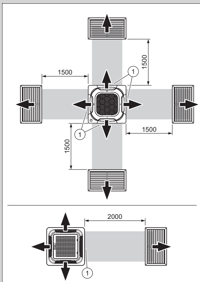
1 Forsku­dt luftudtag
