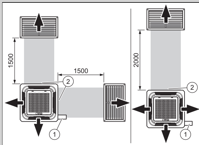
1 Indsugningsluftindtag 2 Forsku­dt luftudtag
