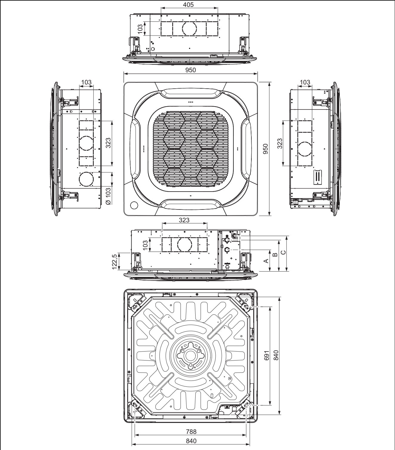
Abmessungen [mm]
