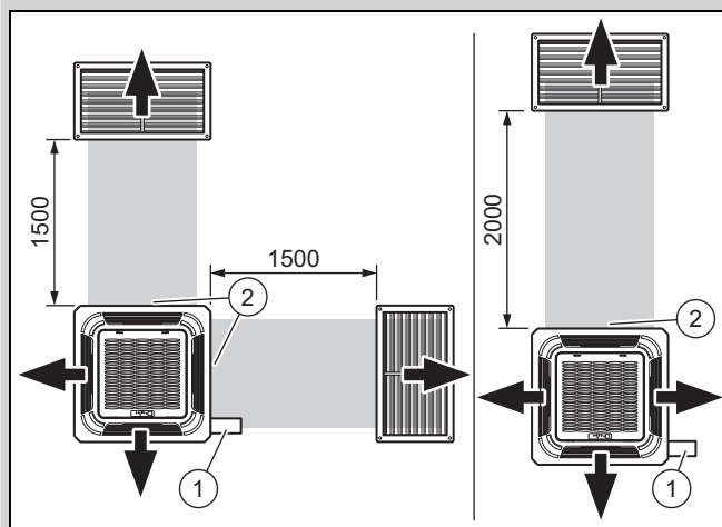
1 Entrée de l'alimentation en air 2 Sortie d'air décalée
