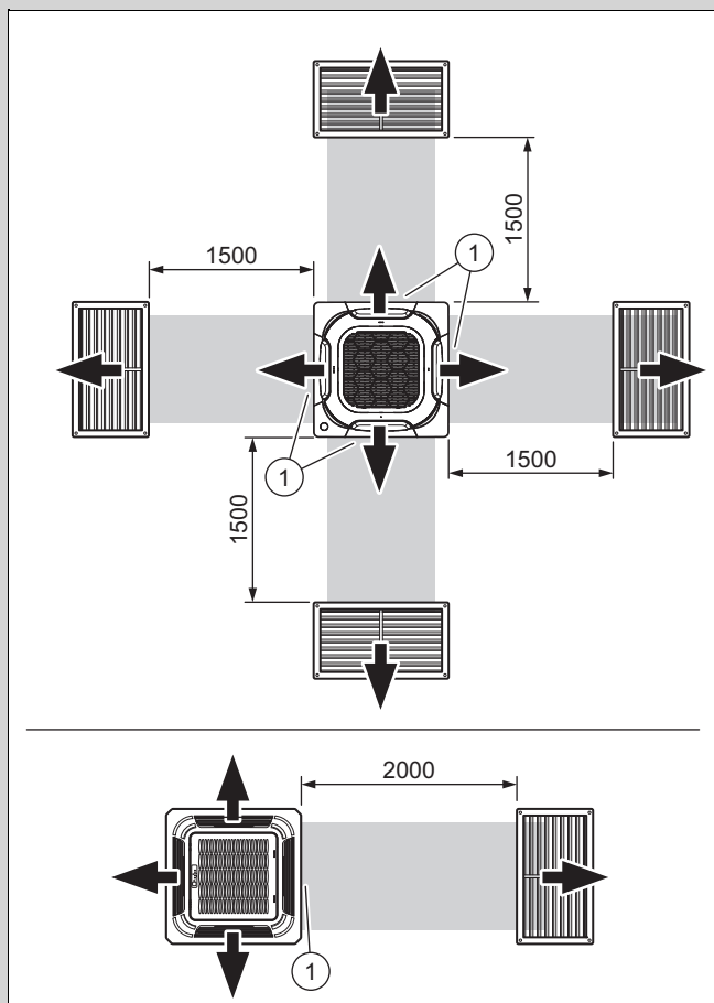
1 Forskjøvet luftutløp
