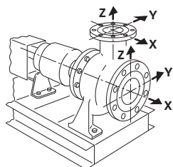
Fig. 8: Lastfall 1A
