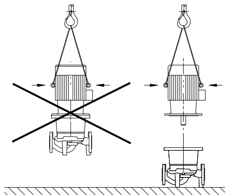
Fig. 2: Transport av motorn
