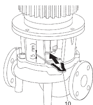
Fig. 17: Placering av montagegaffel
