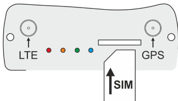
Figur 1 – Montera SIM-kort
