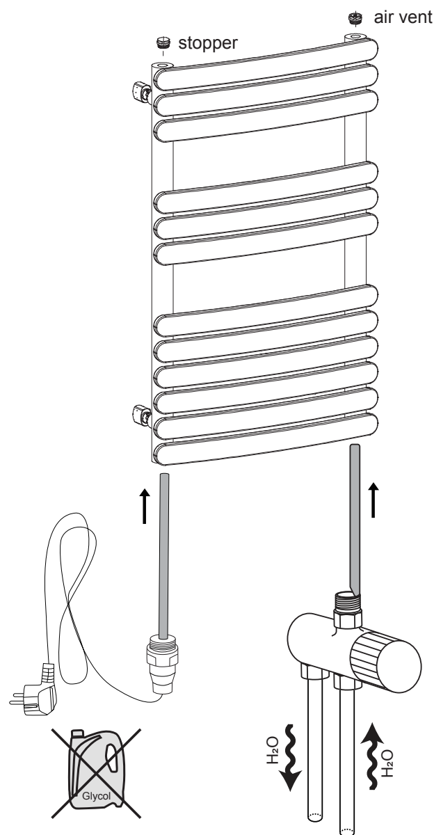
D4 (UK) Combination of electrics system and closed heating (SE) Kombination av elpatron och slutet värmesystem
