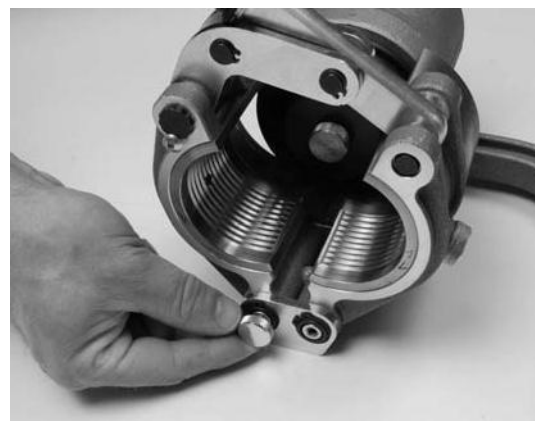
Dra åt den främre fingerskruven för hand. Uppkragningsverktyget är klart för an- vändning.
