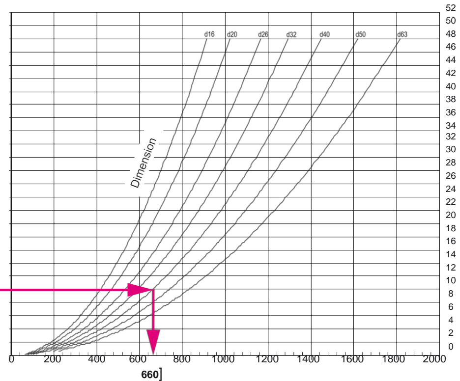
Bestämning av expansionssektionenslängd
