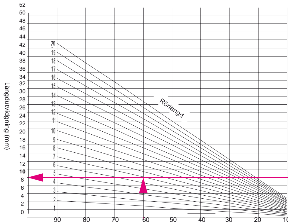
Linjär förändring pga temperaturen i Sanipex MT®-rör
