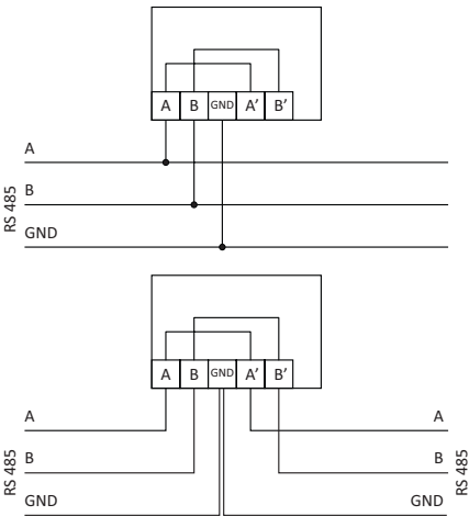
RS 485-kort tillval BACnet MS/TP, Modbus/RTU
