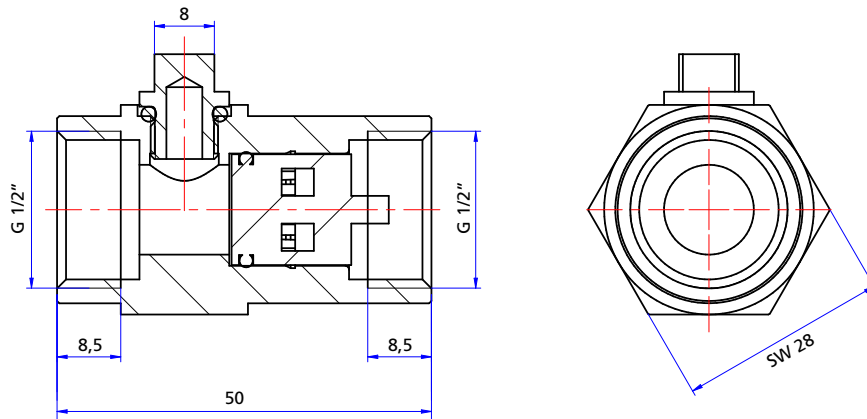
Måttskiss (mm)
