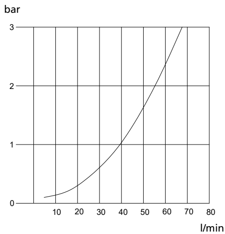
Tryckfall
