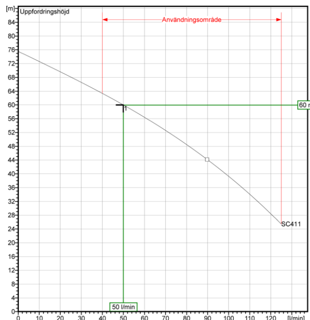
Kapacitetskurva pump SC411T 1,1 kW, 380-415V, 50Hz, 2,8A
