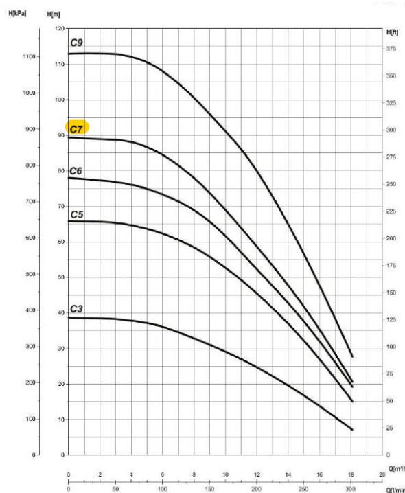
Kapacitetskurva pump SAER C/7 MBS 3,3 kW, 380-415V, 50Hz, 7,2A
