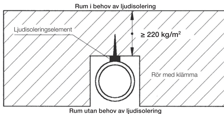
Montering med ljudisoleringselement (FIGUR 27)
