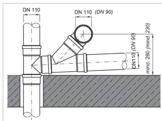
Monteringssituation med standardgrenrör (FIGUR 56)
