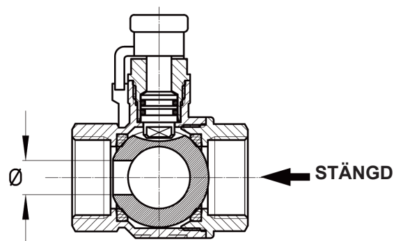
Kula med expansionshål. Pilen visar expansionsriktningen när ventilen är stängd.
