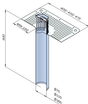
Måttskiss för Takbrunn FURO 180
