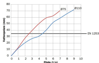
FLÖDESDIAGRAM FÖR TAKBRUNN FURO 180:
