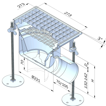
Mått för golvbrunn FURO 105
