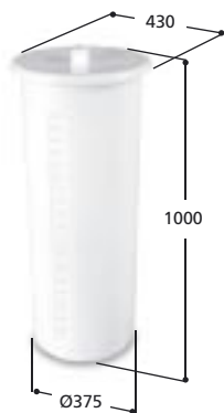
Volym 110 liter Art. nr 10110, vikt 7,5 kg
