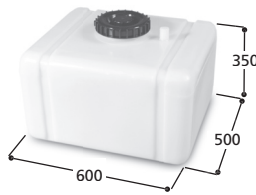
Volym 95 liter Art. nr 20095, vikt 7,5 kg Med Ø 150 mm skruvlock
