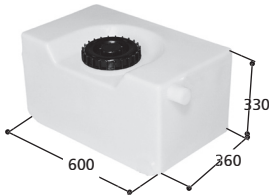
Volym 60 liter Art. nr 20061, vikt 5,5 kg Med Ø 150 mm skruvlock
