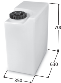
Volym 140 liter Art. nr 20141, vikt 11,0 kg Med Ø 150 mm skruvlock
