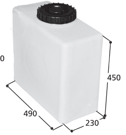
Volym 45 liter Art. nr 20045 vikt 4 kg Med Ø 150 mm skruvlock
