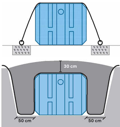
Exempel på förankring i betong eller berggrund.
