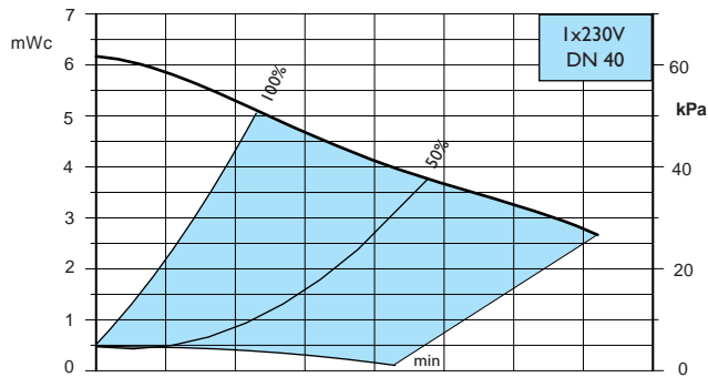
Calio 40-60, ECO
