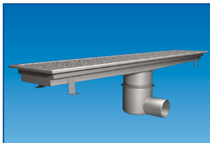
Påbyggnadsdel*. Om 5 dl silkorg eller sandfång väljs som tillbehör till golv- rännan, krävs en påbyggnadsdel.
