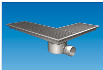
FURO 119-låg = överdel djup 70 mm (tät- fläns till golvtyp klinker K1 placeras på underdelen lika FURO 115). Max längd 1000 mm.
