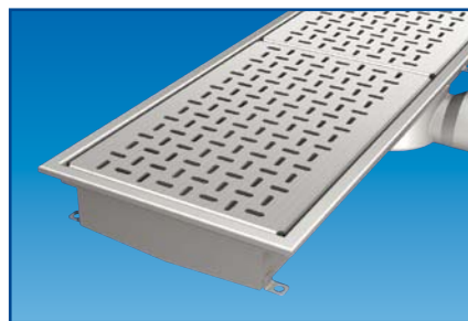
FURO-silplåt med rak mönstring. Belastningsklass K3 eller L15.
