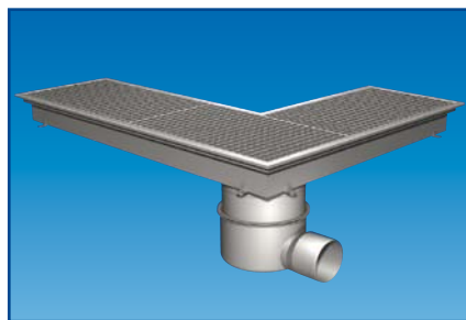
Påbyggnadsdel*. Om 2,7 L silkorg eller 1,5 L sandfång väljs som tillbehör till vinkelrännan, krävs en påbyggnadsdel.
