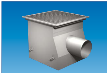
Utlopp Ø 125 mm.
