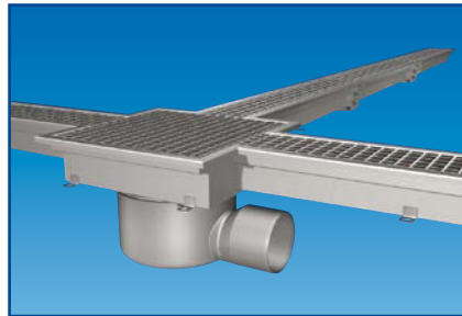
Rännor som ansluter mot utloppsdelens från två, tre eller fyra sidor (ange mått L2, L3 och L4).
