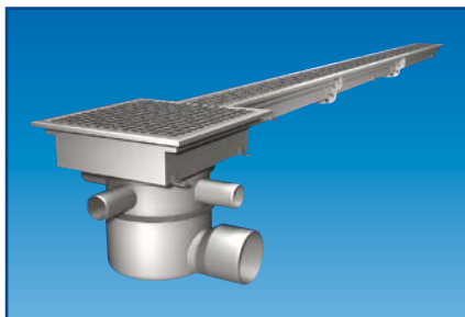
Inloppsdel med ett eller flera inlopp Ø 50 mm slätstos (Ø 40 mm i liten utloppsdel).
