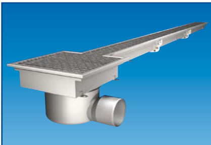
Lamellgaller. Belastningsklass M125.
