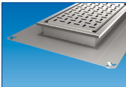
Dräneringshål vid tätskiktsflänsar på brunnar för klinker K1, K4 och K5. (Ett alternativ till dräneringshål kan vara att lägga värmeslingor i golvet som torkar upp den fukt som annars kan bli stående mellan plattor och tätskikt.)
