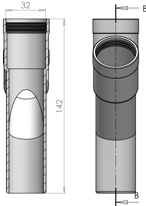
SECTION A-A SCALE 1 : 1.5
