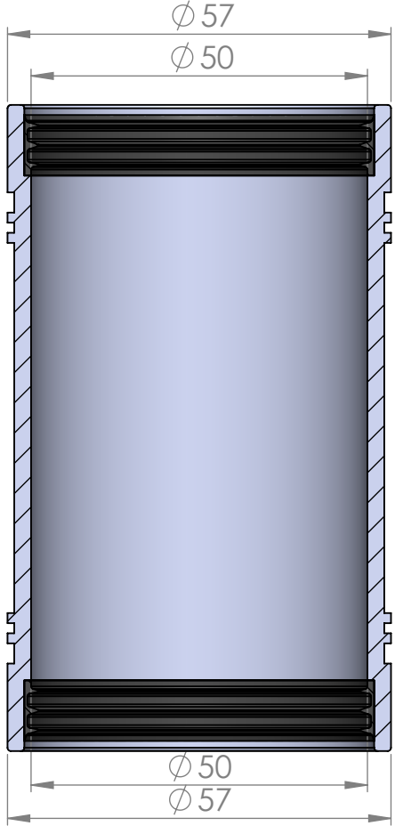
SECTION A-A
