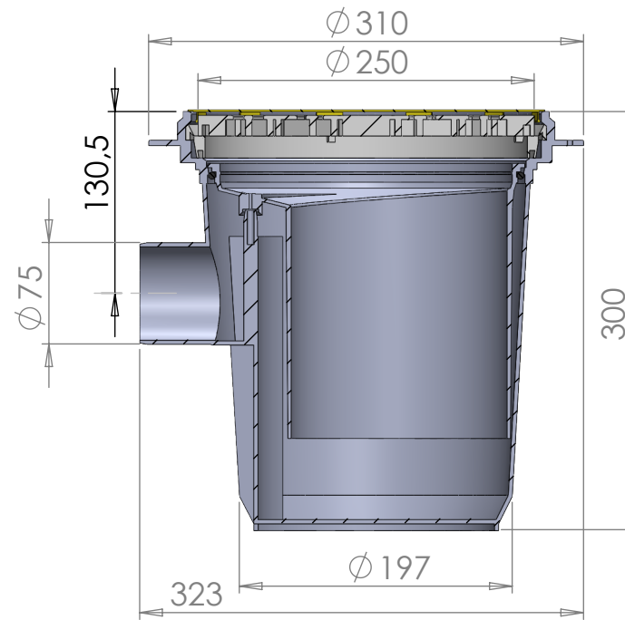
SECTION A-A SCALE 1 : 5
