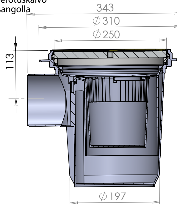
SECTION A-A SCALE 1 : 5
