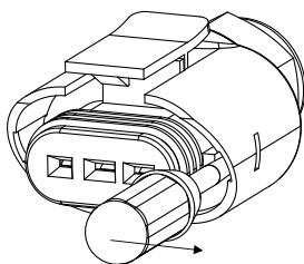
Bild 15: Demontera kontakten
