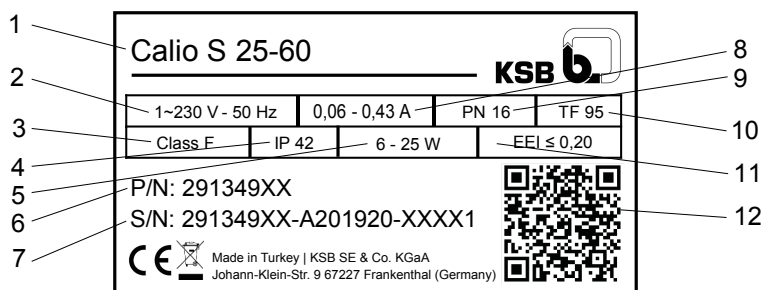
Bild 1: Märkskylt (exempel)
