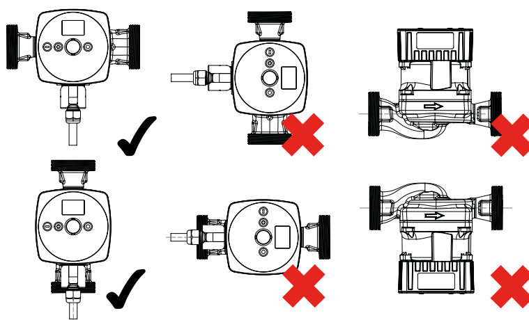
Bild 3: Tillåtna monteringslägen
