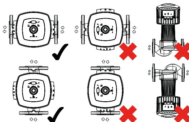
Bild 7: Tillåtna monteringslägen
