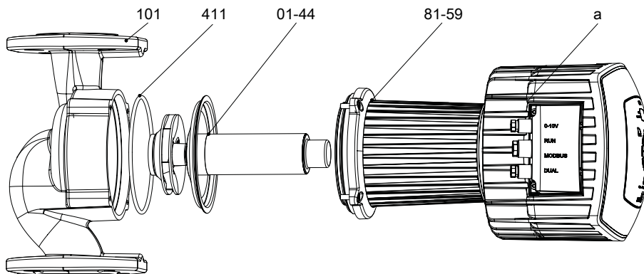
Bild 29: Sprängskiss
