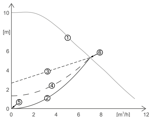
Bild 23: Eco-mode och proportionellt tryck med modellstorlek 25-100 som exempel
