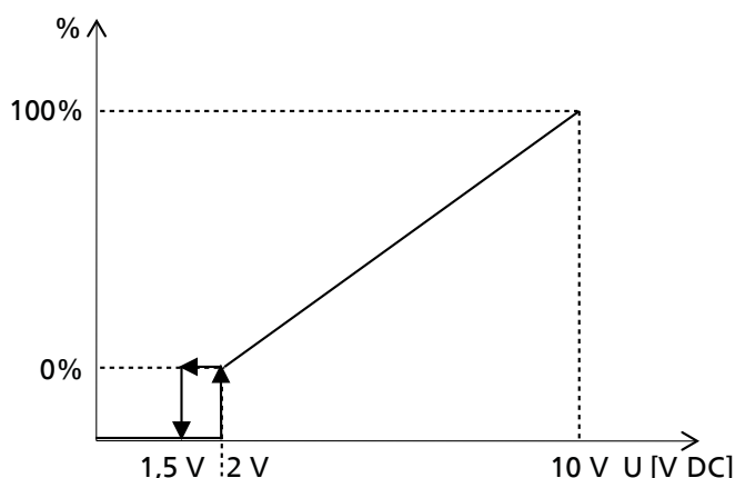
Bild 27: Analog signal 0-10 V som börvärdesinställning på pumpaggregatet
