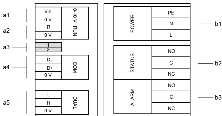
Bild 30: Elektriskt anslutningschema
