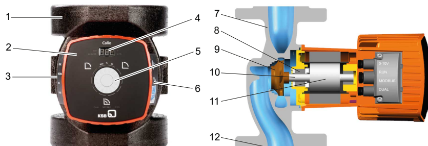
Bild 5: Beskrivning och sprängskiss av pumpaggregatet
