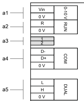
Bild 16: Plintschema dubbelpumpdrift
