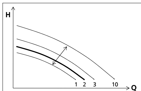
Bild 25: Funktion termostatdrift, drift på varvtalssteg 2
