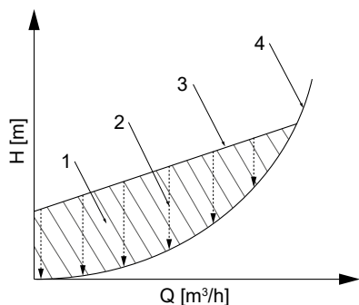
Bild 28: Den dynamiska styrningens princip
