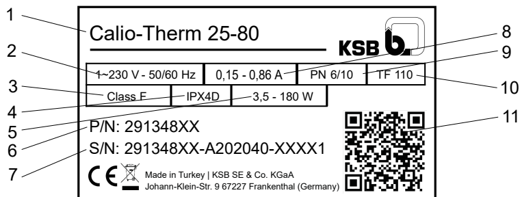
Bild 4: Märkskylt (exempel)
