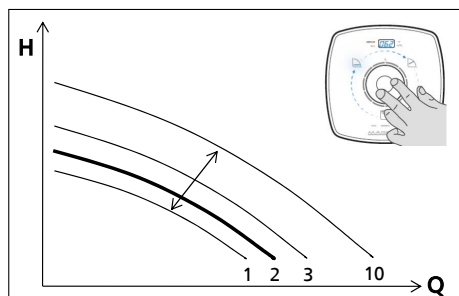
Bild 26: Inställning termostatdrift
