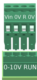
Bild 12: Plintpar RUN
