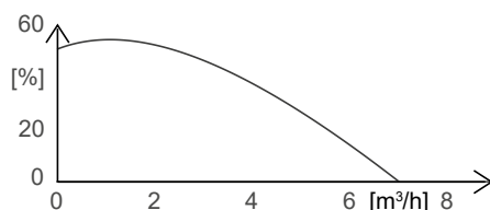
Bild 24: Besparingspotential för Eco-Mode jämfört med proportionellt tryck med modellstorlek 25-100 som exempel
