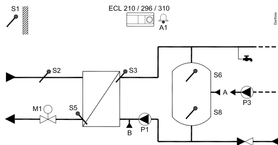
Vanlig A217.1-/A317.1-applikation:
