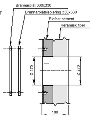
Fig. 12 - Anvisning för borrning av lucka TRIO 1100-1320
