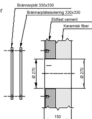
Fig. 10 - Anvisning för borring av lucka TRIO 840
