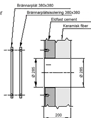
Fig. 13 - Anvisning för borrning av lucka TRIO 1600-1900
