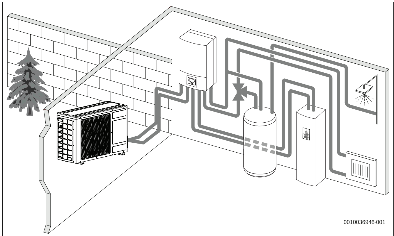
Bild 2 Värmepump för uteenhet, inneenhet AWS B utan eltillskott, extern varmvattenberedare och extern extra värmekälla
