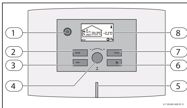
Bild 3 Kontrollpanelen
