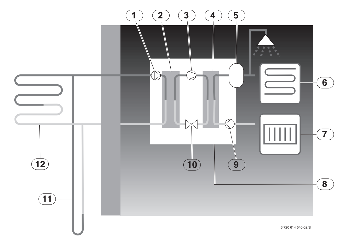
Bild 2 Funktionsbeskrivning
