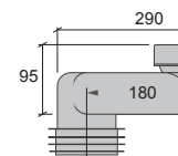
A + K2 WC - Stos Offset 180 Excentrisk 180 mm RSK 310 66 81 NRF 619 66 56
