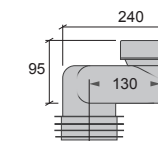
A + K2 WC - Stos Offset 130 Excentrisk 130 mm RSK 310 66 80 NRF 619 66 55
