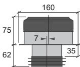
A GAS - WC 7 Utan huv, Excentrisk 7 mm RSK 310 67 03 NRF 56 884 21
