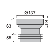
A WC - Stos, Centrisk RSK 310 66 84 NRF 619 66 72
