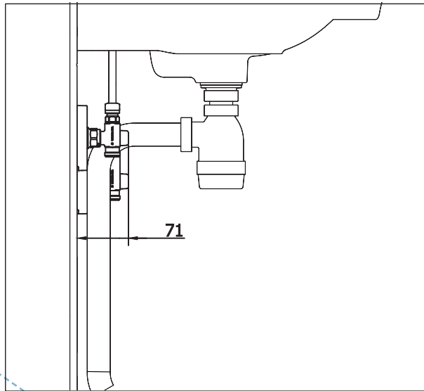
Sidovy
