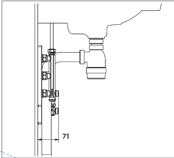
Sidovy
