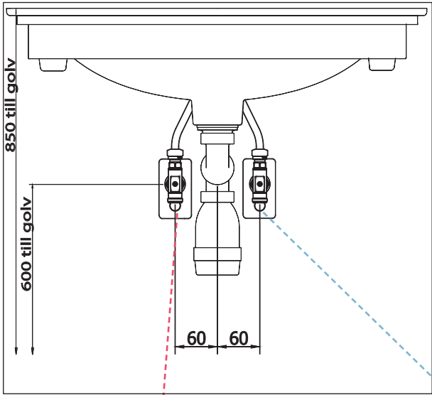
Frontvy
