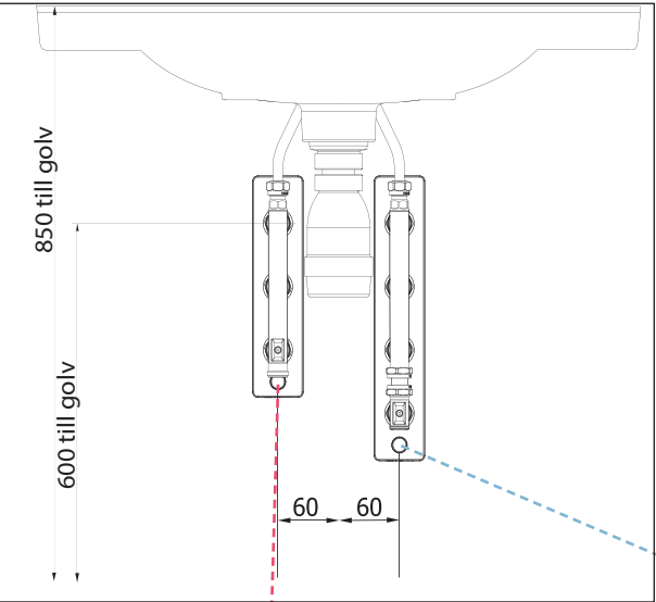
Frontvy
